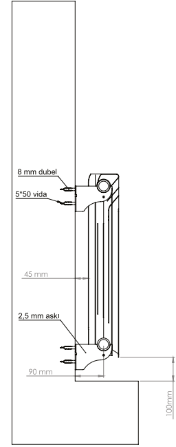
NF 500 ULTRA DUVARA MONTAJ DETAYI
